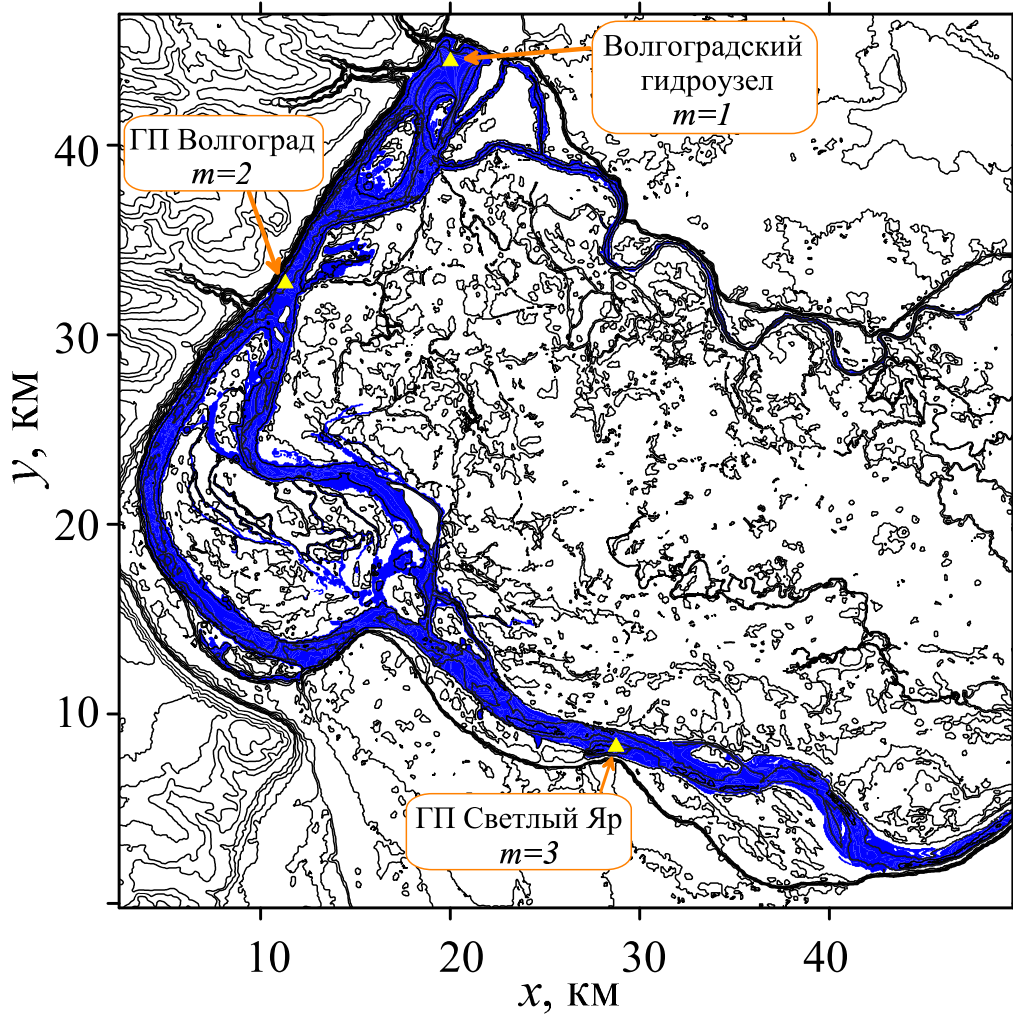
Рис. 2. Цифровая модель северной части ВАП. Показаны положения гидропостов, изолинии рельефа, распределения воды в ВАП накануне весеннего пуща воды (синий цвет). Ось y направлена на север
