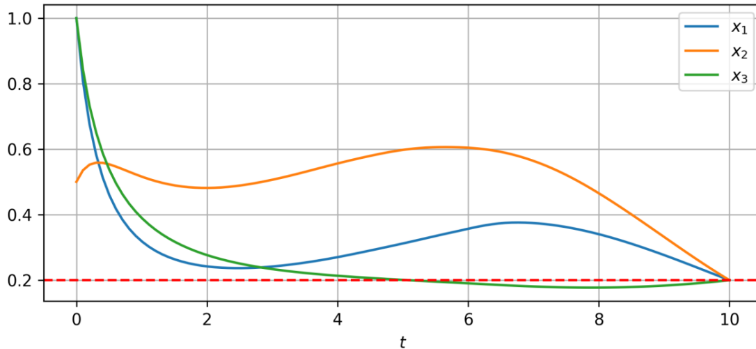
Рис. 4. Траектории системы (1) для R_1(-0.54295917, 0.08043992, 0.00126864) , R_2(1.14936551, -0.35249694, 0.04373466) , R_3(0.8862529, -0.09851022, 0.00590944) с использованием алгоритма Пауэлла
