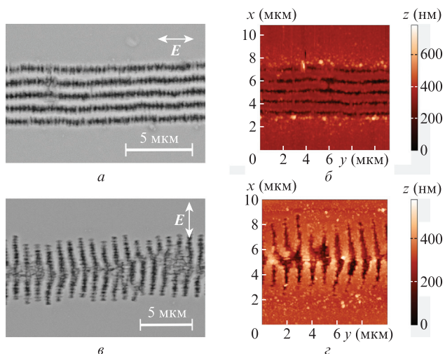
Рис.4. СЭМ-изображения ТЛИППС, сформированных на поверхности нихрома (80/20) лазерным излучением с W = 83 нДж и направлениями поляризации излучения параллельно (а) и перпендикулярно (в) направлению сканирования, а также соответствующие АСМ-изображения (б, г).
