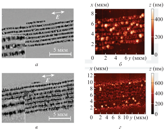
Рис.3. СЭМ-изображения ТЛИППС, сформированных на поверхности хрома лазерным излучением с W = 83 (а) и 102 нДж (в), а также соответствующие АСМ-изображения (б, г). На вставках на рис.3,а и в приведены увеличенные изображения структуры.
