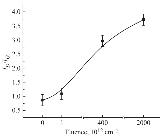
Рис. 2. Зависимость отношения интегральной интенсивности пиков I_D/I_G от флюенса.
