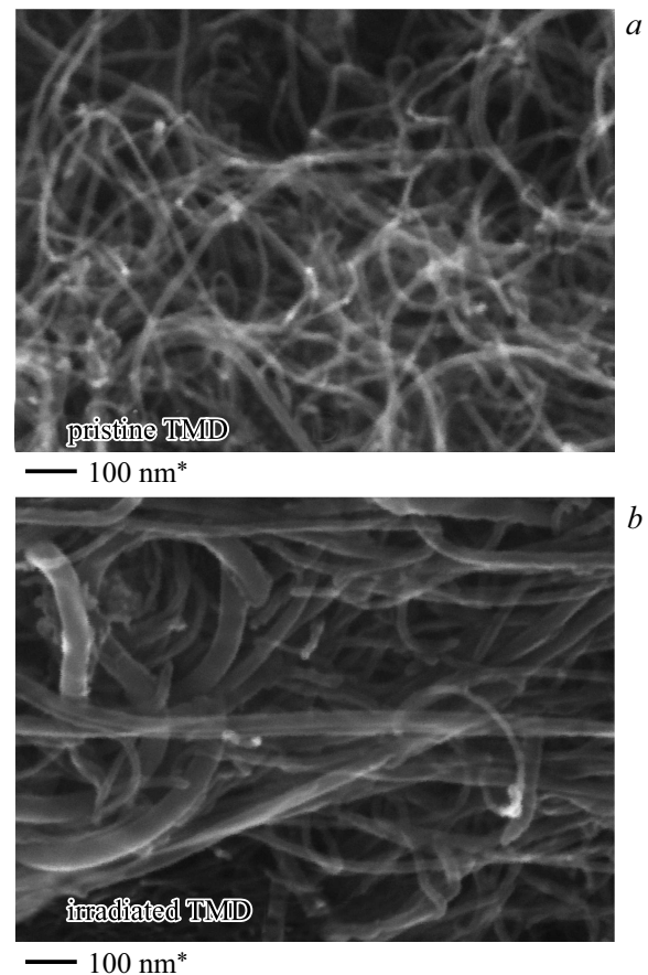
Рис. 3. СЭМ-изображения неoblученного ( a ) и облученного флюенсом 2 \cdot 10^{15} \text{ см}^{-2} ( b ) образцов МУНТ ТМД.
