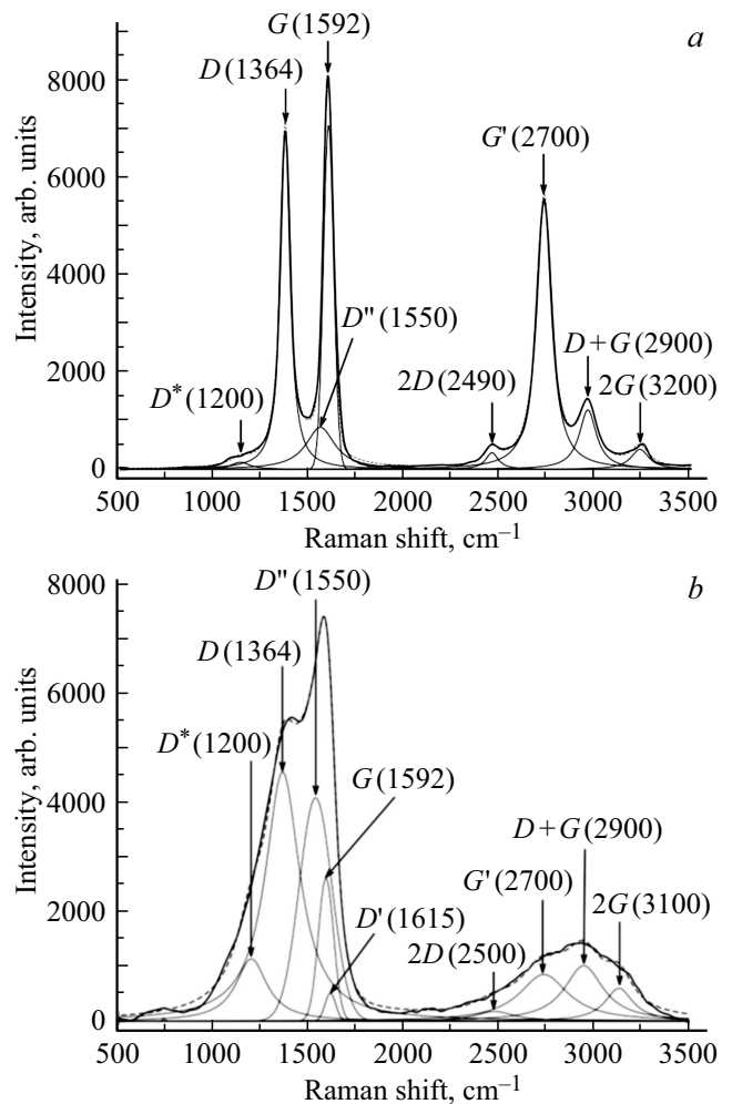
Рис. 1. Спектры КРС МУНТ и их разложение: a — необлученные МУНТ ТМД, b — облученные флюенсом 2 \cdot 10^{15} \text{см}^{-2} .
