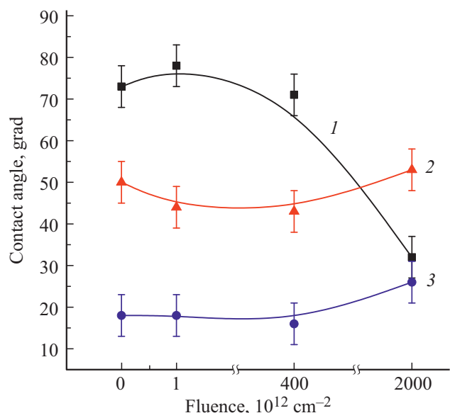
Рис. 5. Зависимость угла смачиваемости образцов МУНТ ТМД от флюенса для дистиллированной воды (1), этиленгликоля (2), циклогексана (3).
