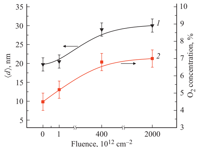
Рис. 4. Зависимости от флюенса: среднего диаметра МУНТ ТМД (1) и концентрации \text{O}_2 в образцах МУНТ ТМД (2).
