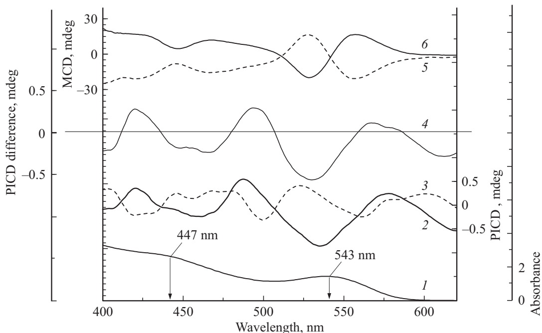
Спектры МКД и спектры ФИКД квантовых точек CdSe/ZnS в хлороформе: 1 — спектр поглощения; 2 — спектр ФИКД, полученный после 40 минут облучения светом с левой круговой поляризацией; 3 — спектр ФИКД, полученный после 40 min облучения светом с правой круговой поляризацией; 4 — разностный спектр ФИКД (ФИКД, полученный после 40 минут облучения светом с левой круговой поляризацией, минус ФИКД, полученный после 40 минут облучения светом с правой круговой поляризацией); 5 — спектр МКД при H = +1.5 T; 6 — спектр МКД при H = -1.5 T.
