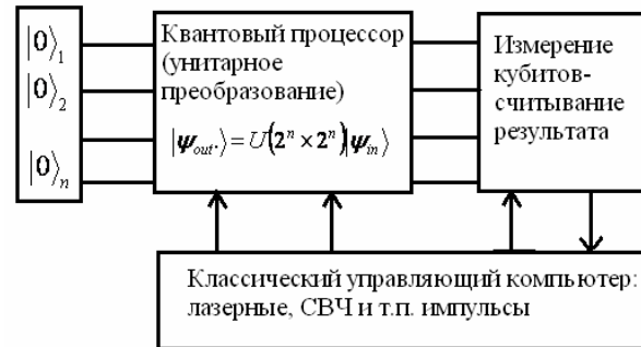
Рис. 5. Блок-схема идеального квантового компьютера
