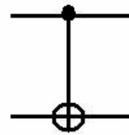
Рис. 4. Графическое изображение двухкубитового элемента CNOT
