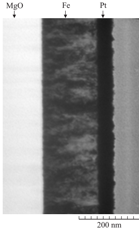
Рис. 1. Поперечный разрез исходного двухслойного образца Fe_{87}Pt_{13} .
