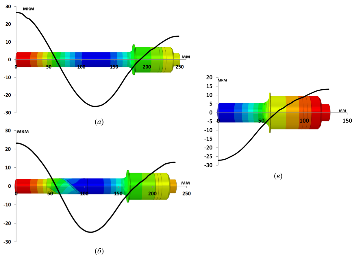
Рис. 11. Распределение амплитуды колебания продольной волны волнового преобразователя с концентратором продольно-крутильных колебаний с непостоянным поперечным сечением из-за наличия винтовых канавок (а), волнового преобразователя с концентратором с поперечным сечением в виде круга (б) и 1/2-волнового преобразователя с концентратором с поперечным сечением в виде круга (в)
