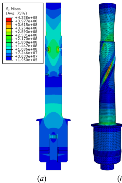
Рис. 14. Распределение интенсивности напряжений по Мизесу по сечению (а) и на поверхности (б)
