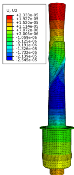
Рис. 12. Распределение амплитуд продольных колебаний
